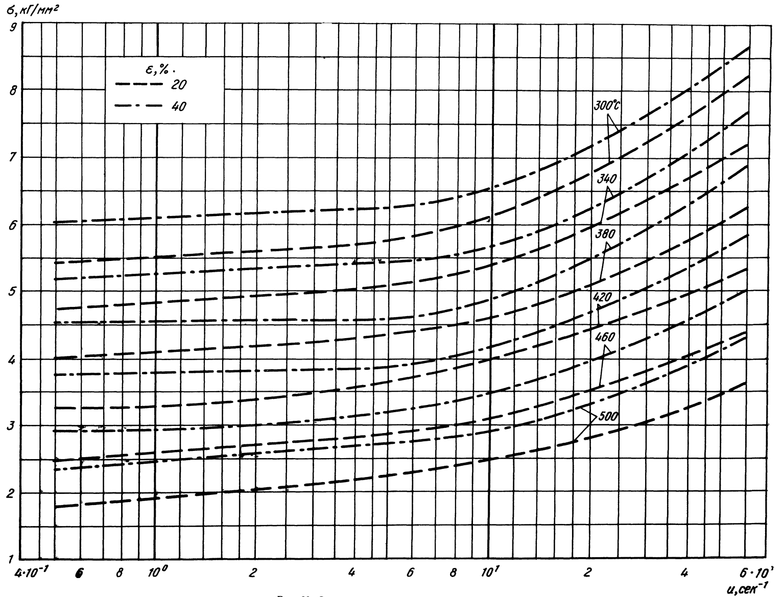
Рис 36 Сопротивление деформации алюминия АД
