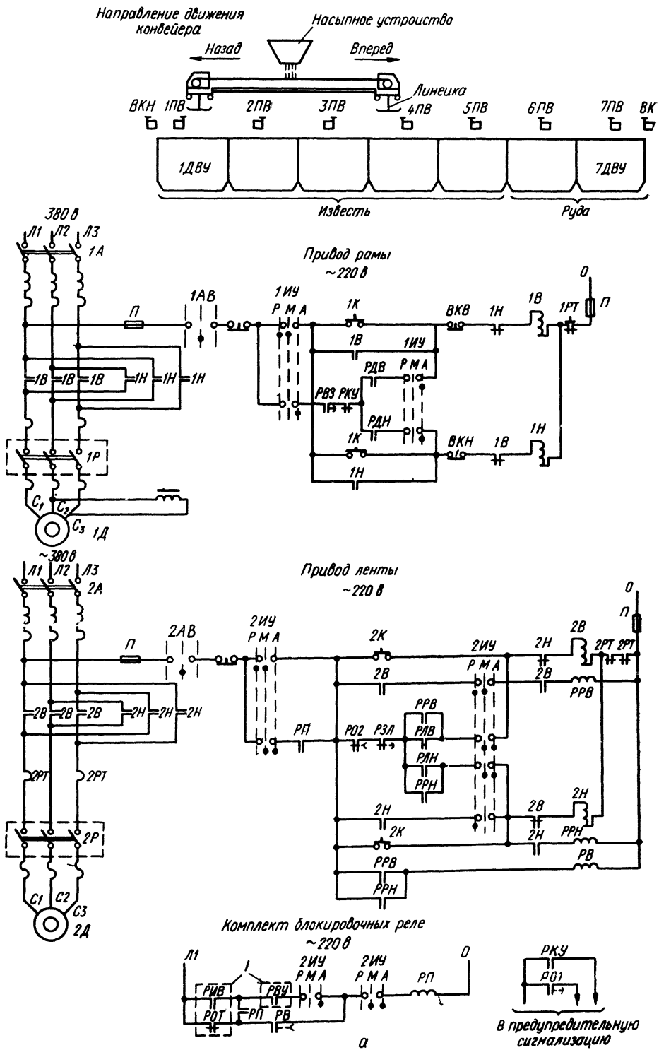
Рис 114 Схема управления передвижным конвейером I — из пускового комплекта схемы управления поточным производством; II — контакты датчиков
