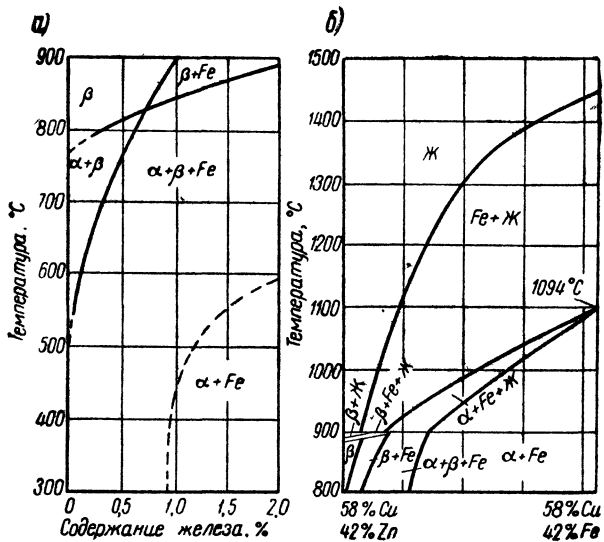
Рис. 145. Вертикальные разрезы диаграммы фазового равновесия системы медь — цинк — железо:
