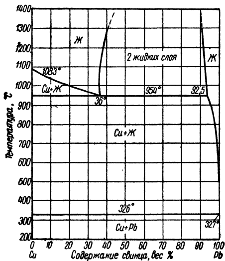
Рис. 146. Диаграмма фазового равновесия медь — свинец
