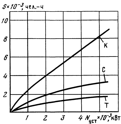
Рис. 4.2. График зависимости трудоемкости S ремонтов электрооборудования от установленной мощности N_{уст} приводов
